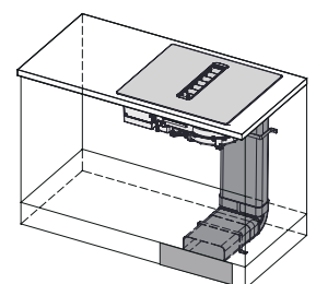
Instalación de salida al cuarto bajo el zócalo
