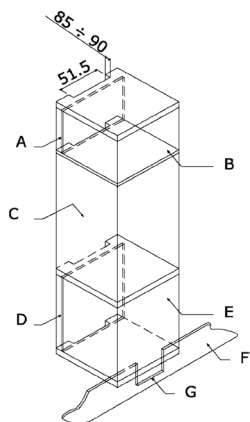
Рис. 8: Требования к вентиляции и зазорам при установке простой электрической духовки в верхнем шкафу.
